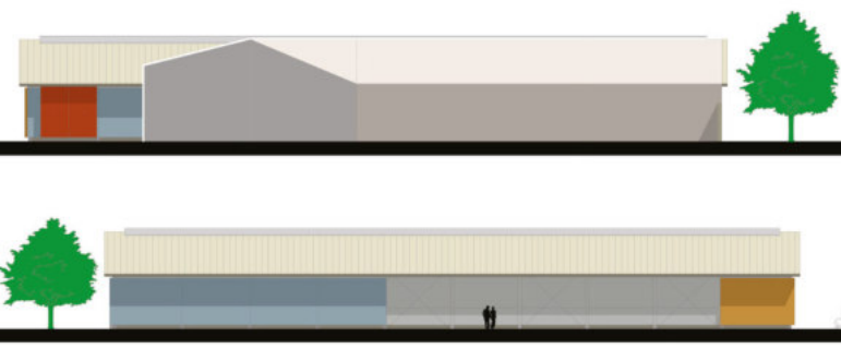
Neubau einer Bewegungshalle für Pferde, Großjena Vorentwurf - Stahlkonstruktion mit farbiger Blechverkleidung, Belichtungs / Belüftungsfeldern und Oberlichtband
